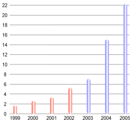
Рис. 2. Рост количества пользователей Интернетом в России с 1999 г. по 2005 г.
