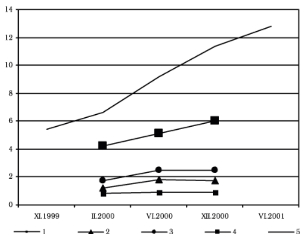
Рис. 1. Динамика изменения количества Интернет-пользователей в России в 1999–2001 гг., млн. человек.*
